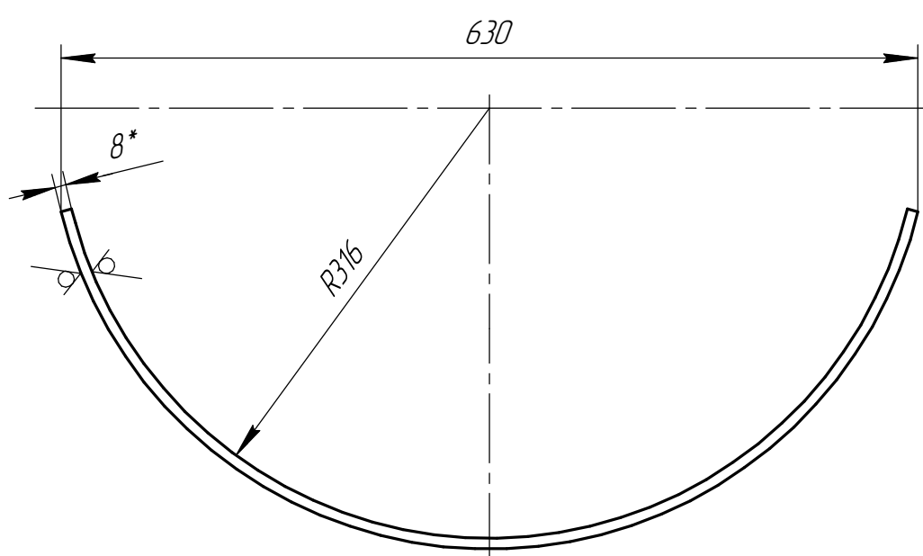
Дет. поз. 3 (1:2,5)
